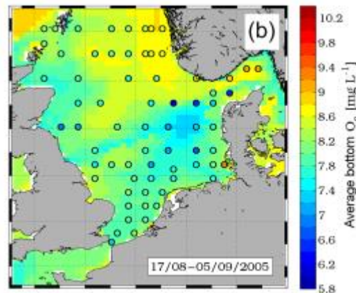
Abb. 10: Darstellung der Sauerstoffverteilung in der Nordsee im August und September 2005. Ausschnitt einer Darstellung von GROßE et al. (2016)
