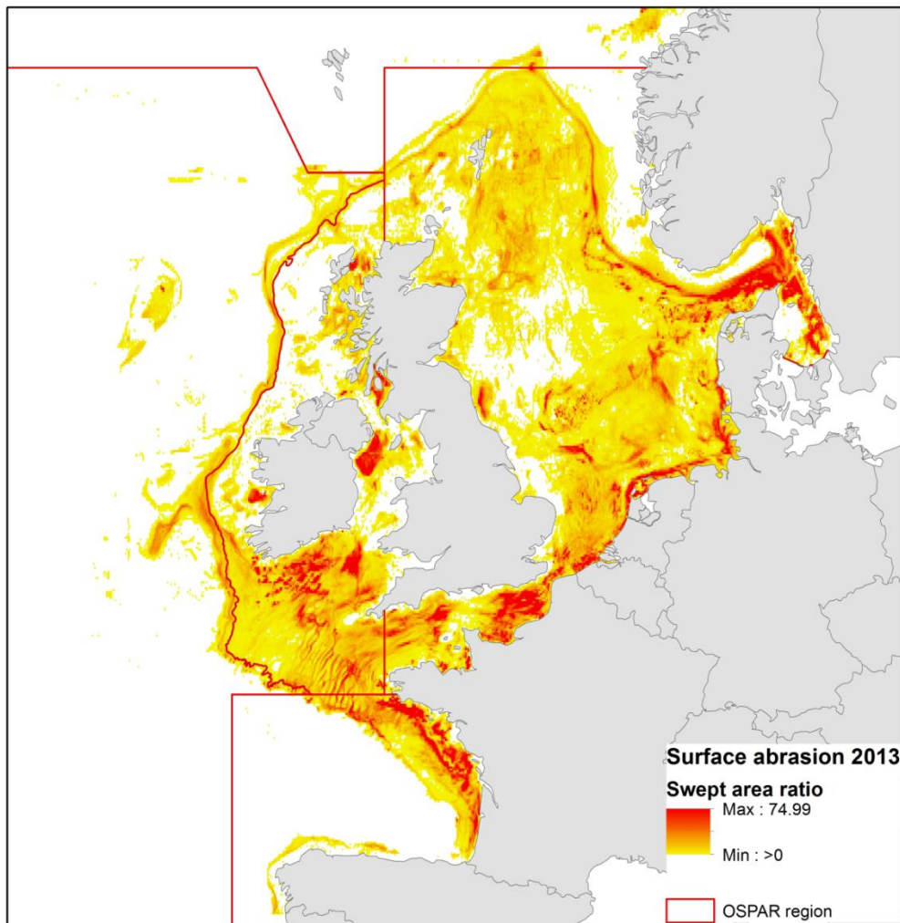
Abb. 18: Intensität der Belastung durch bodenberührende Fischerei auf der Meeresbodenoberfläche 2013
